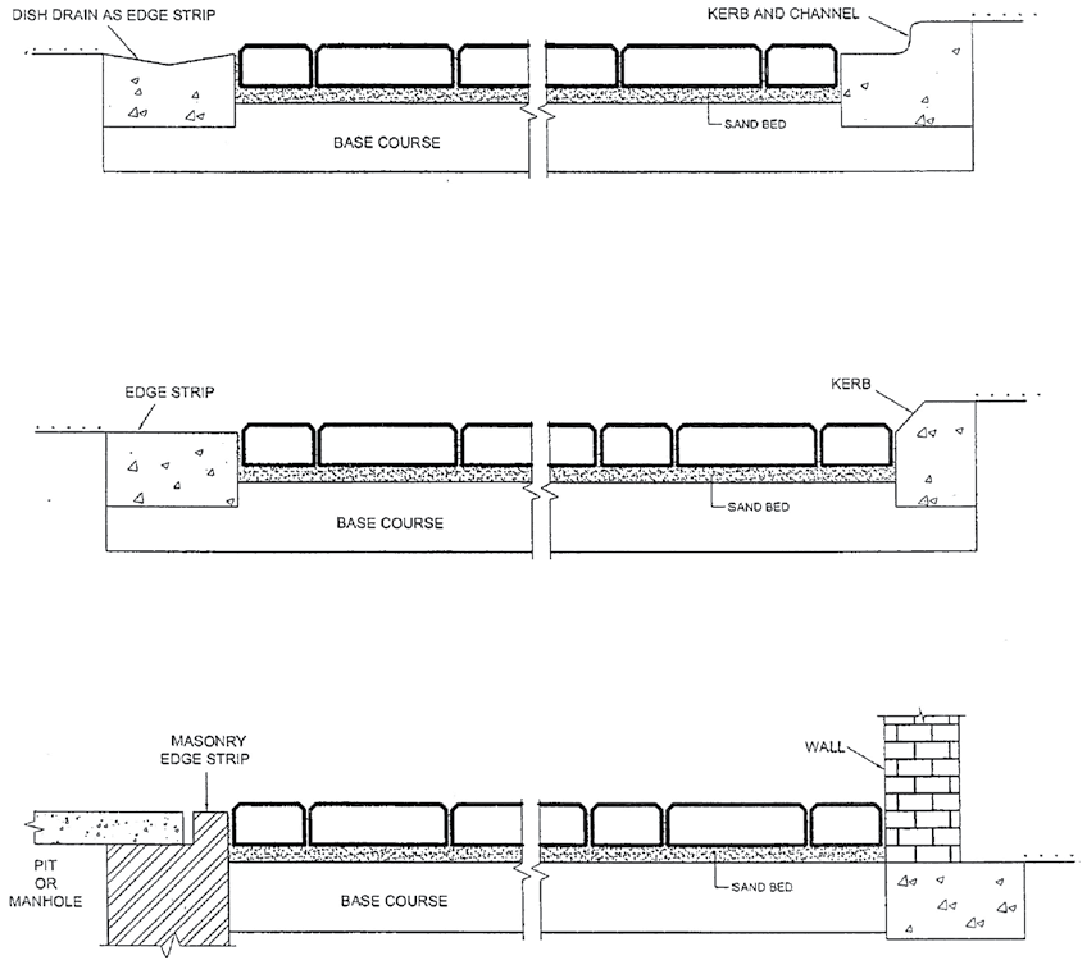
Fig.8 Edge Restraints
