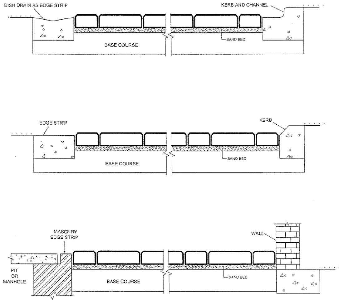
Fig.8 Edge Restraints
